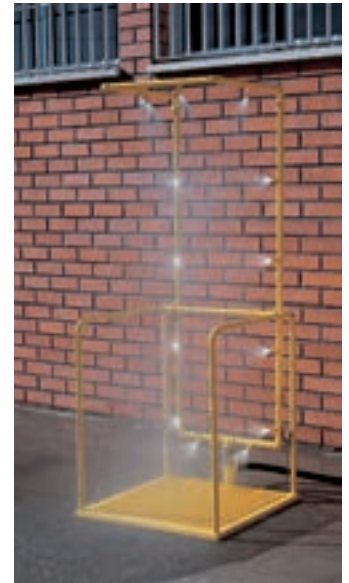
Cabina de descontaminación con 14 rociadores (mod 4810).
